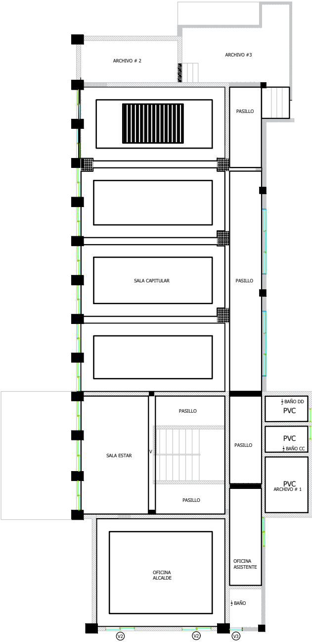
PLANTA TECNICA TECHO FACIA 2DO NIVEL
