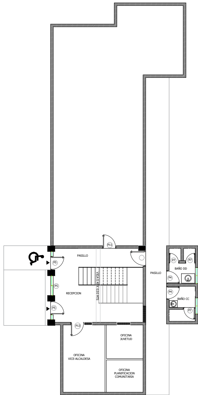
PLANTA TECNICA PUERTAS Y VENTANAS 1ER NIVEL
