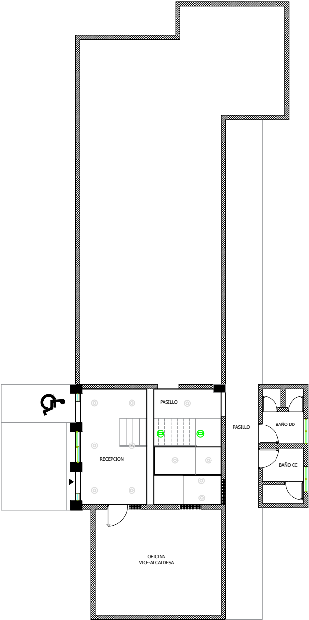
PLANTA TECNICA ILUMINACION 1ER NIVEL
