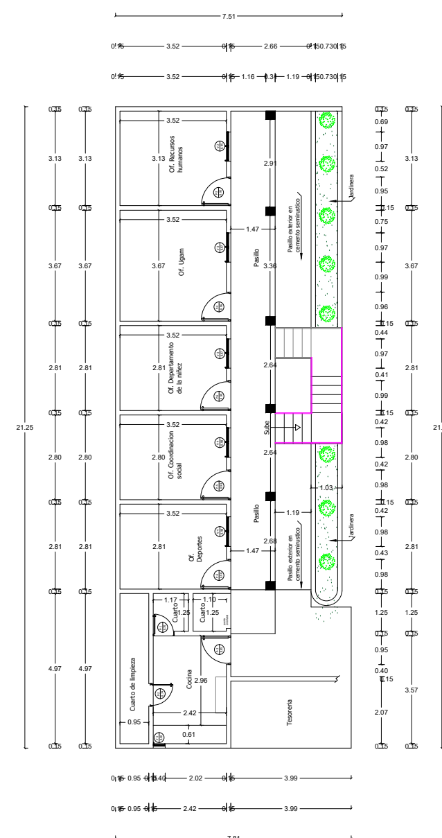
PLANTA DIMENSIONADA PRIMER NIVEL
