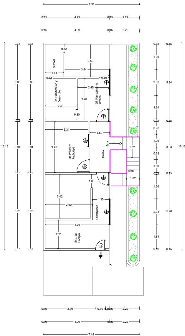
PLANTA DIMENSIONADA SEGUNDO NIVEL
