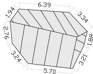
VISTA EN PLANTA DEL PERGOLADO CON SUS DIMENCIONES.
