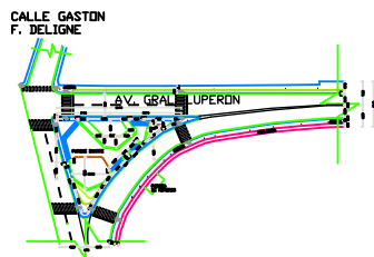
PLANTA DIMENSIONADA
